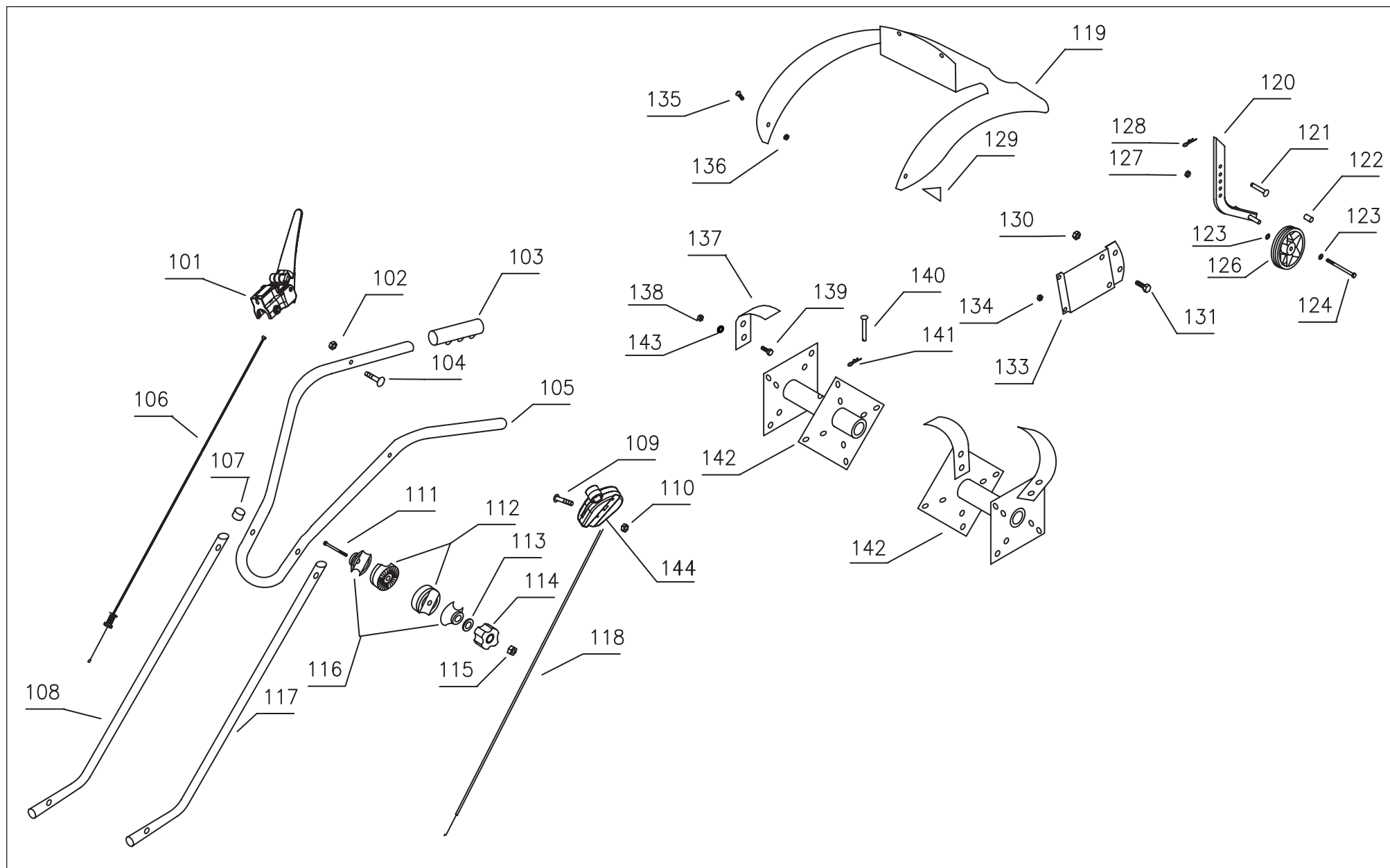
Схема 2. Сборочные единицы и детали
