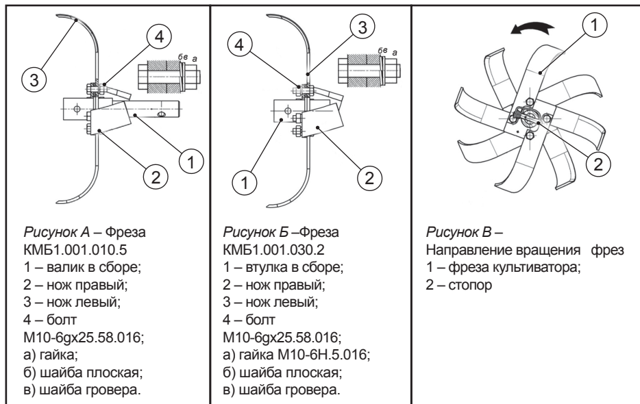
Рис. 3 Схема сборки фрез
