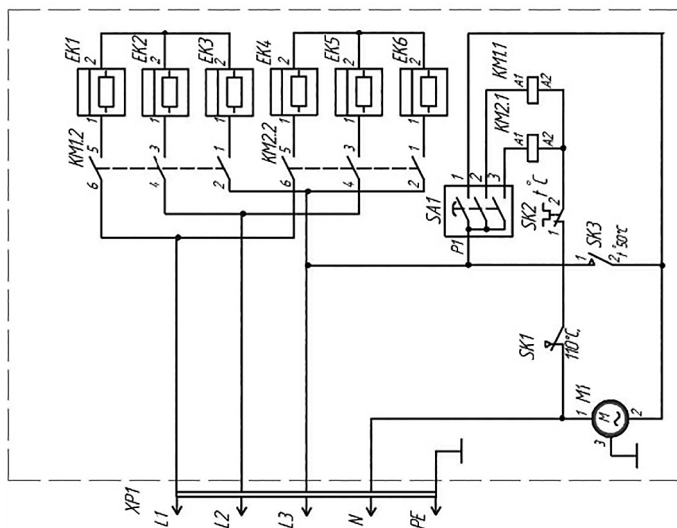
Схема коммутации переключателя SA1
