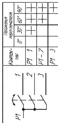
Схема коммутации переключателя SA1
