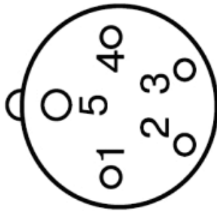
Рис. 4 Схема контактов на вилке
