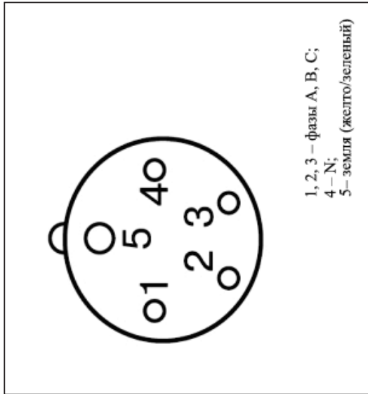
Рис. 4 Схема контактов на вилке
